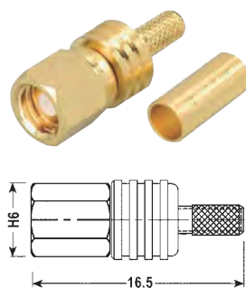
Art. SBC/100 per cavo RG174 50ohm
